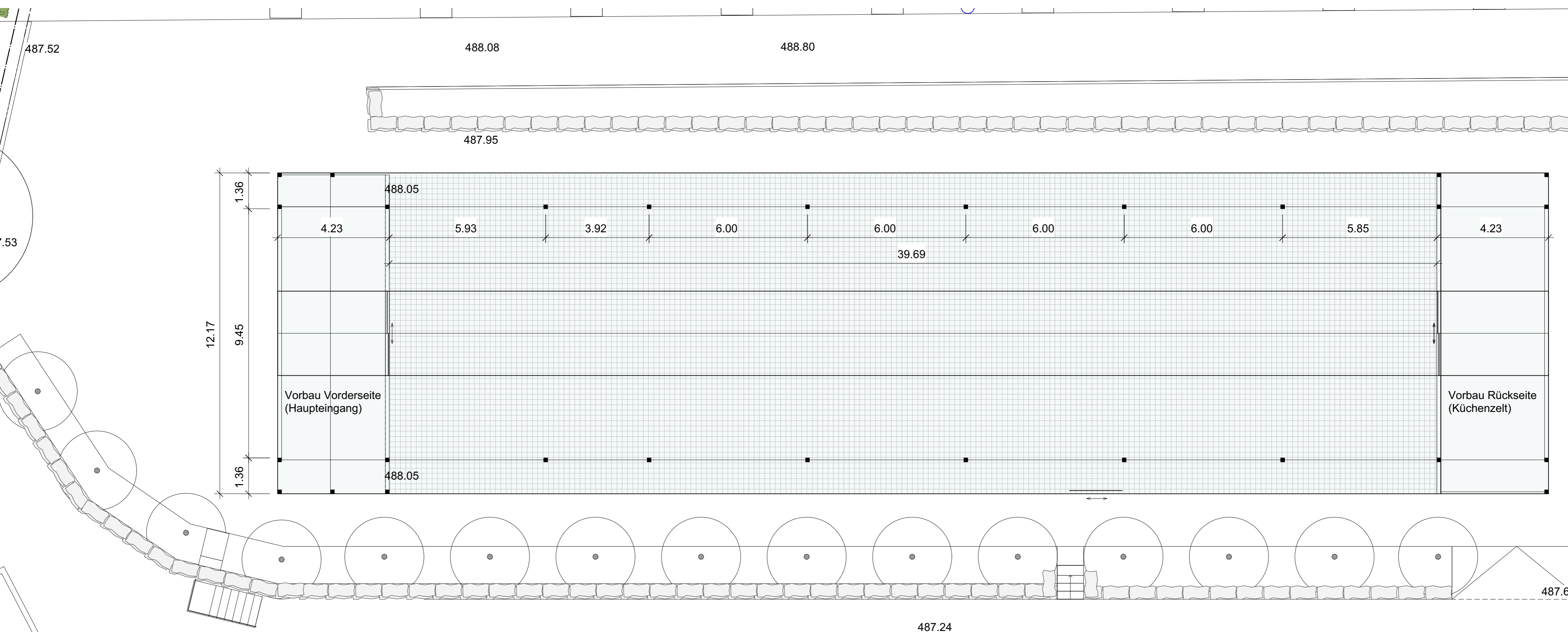
1 Grundriss Glashaus Baumschule Mettmenstetten. Planformat A2 Maßstab: 1:100
